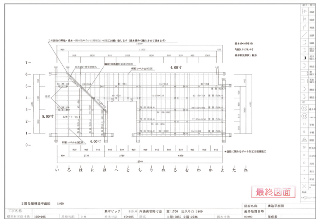
屋根伏図
