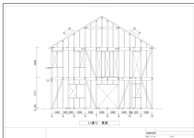
軸組図
