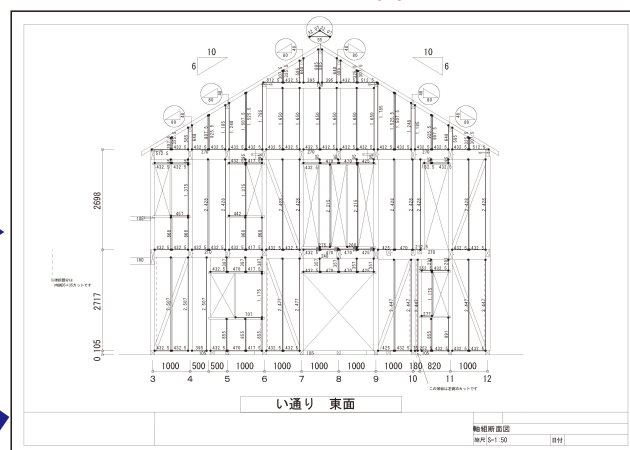
プレカット図
